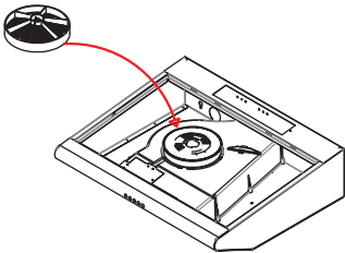
Hapi 2 Vendosni filtrin e karbonit.
