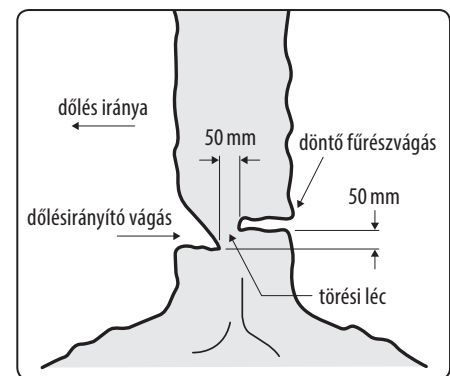
11. ábra. A fadóntás lépései: fűrészelés
